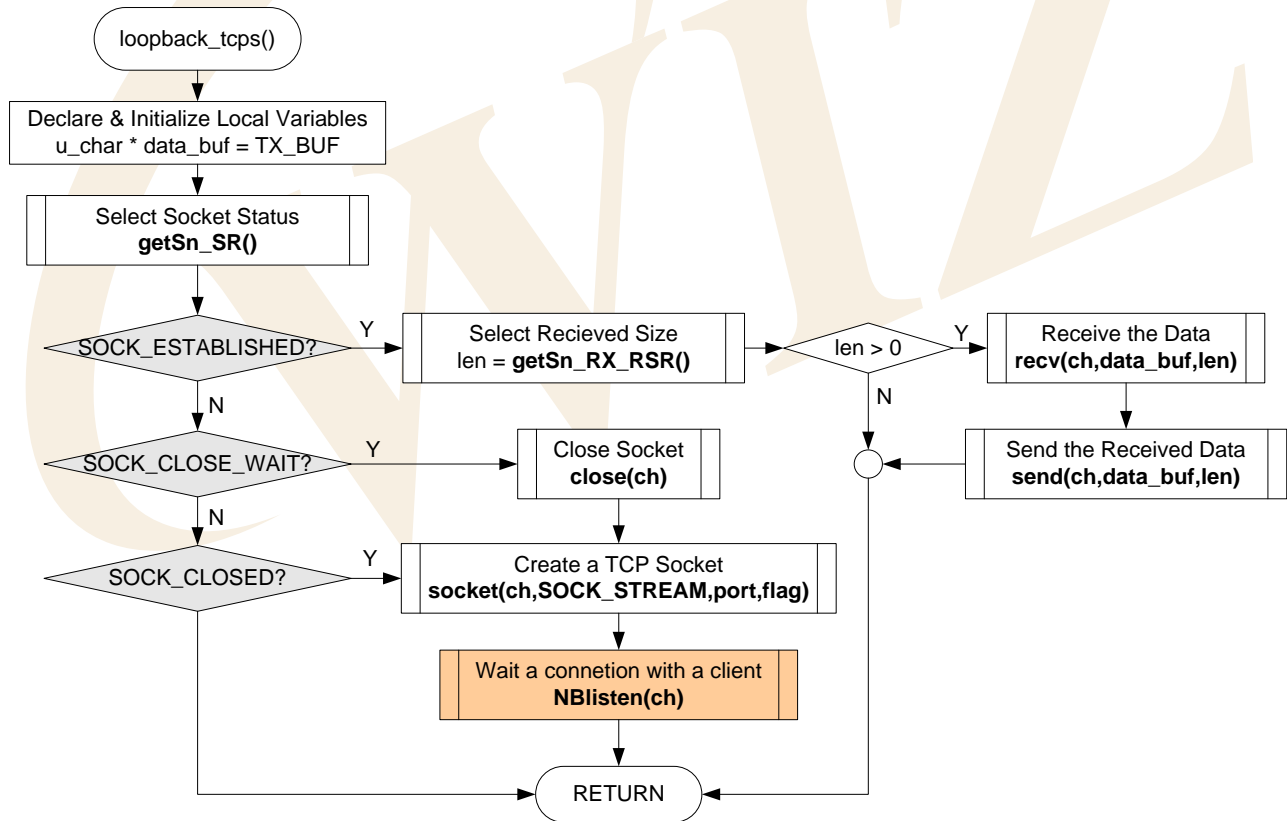
< Fig 3.14 : loopback_tcps() >
