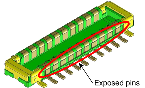
プラグ Plug PN: 505070-**20
