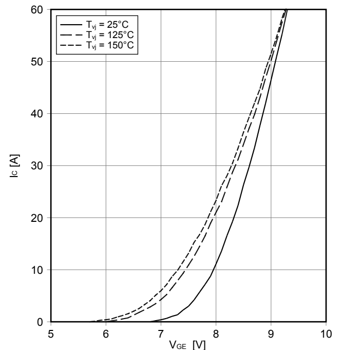
Übertragungscharakteristik IGBT-Chopper (typisch) transfer characteristic IGBT-Chopper (typical) I_C = f(V_{GE}) V_{CE} = 20\text{ V}
